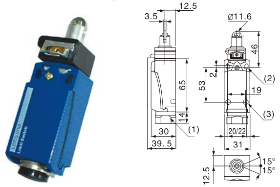
LL3XCDR2127P20 热塑滚轮垂直推杆
