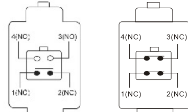
一开一闭型 1NC+1NO Type
